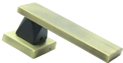
Mars
